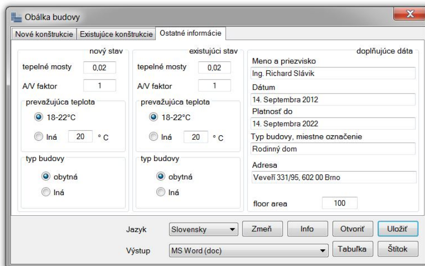
Obrázek 2 Hlavní okno aplikace s rozšiřujícími daty
